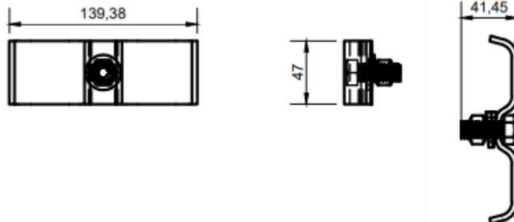
Imagen 02: Dimensiones del Soporte Diseño Especial
