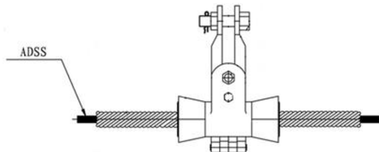
Imagen 02: Grapa Trunion instalada
